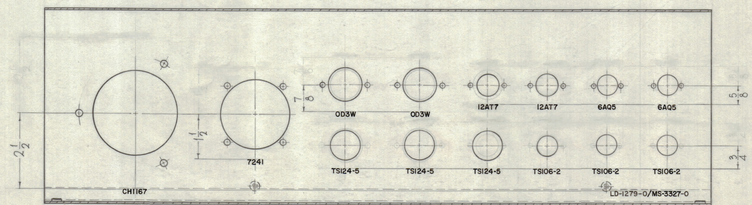
SECTION V-V
